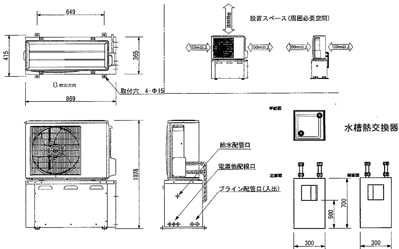
外観寸法図
